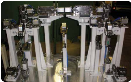
Schweißvorrichtung für die Automobilindustrie
